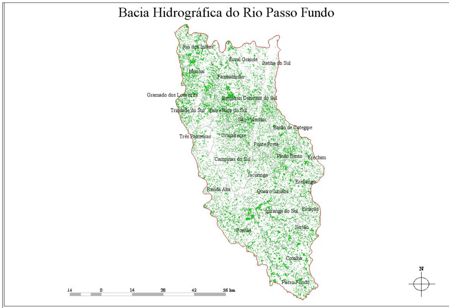
Figura 3: Cobertura de mata nativa na Bacia Hidrográfica do Rio Passo Fundo.
